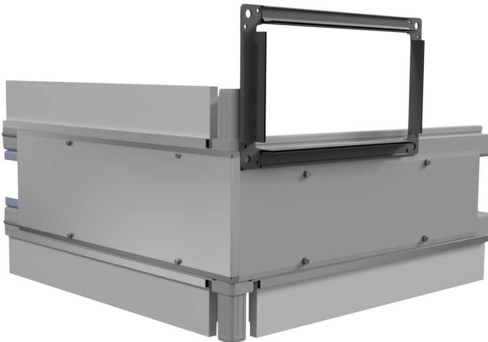
d) Zusammenbau Abdeckblech bei einfacher Anschlussöffnung
